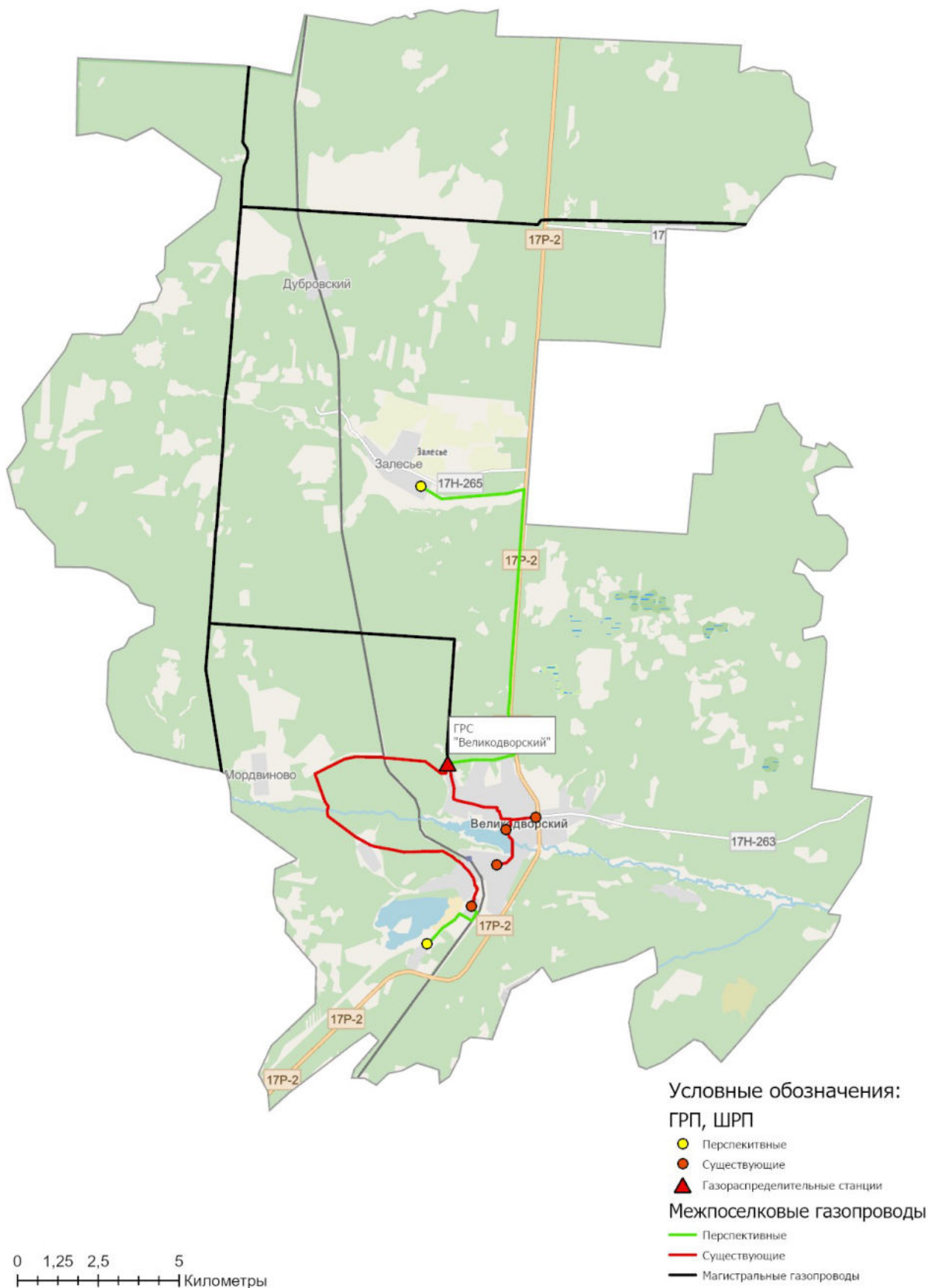
Рисунок 10.6 - Перспективная схема газификации территории муниципального образования
