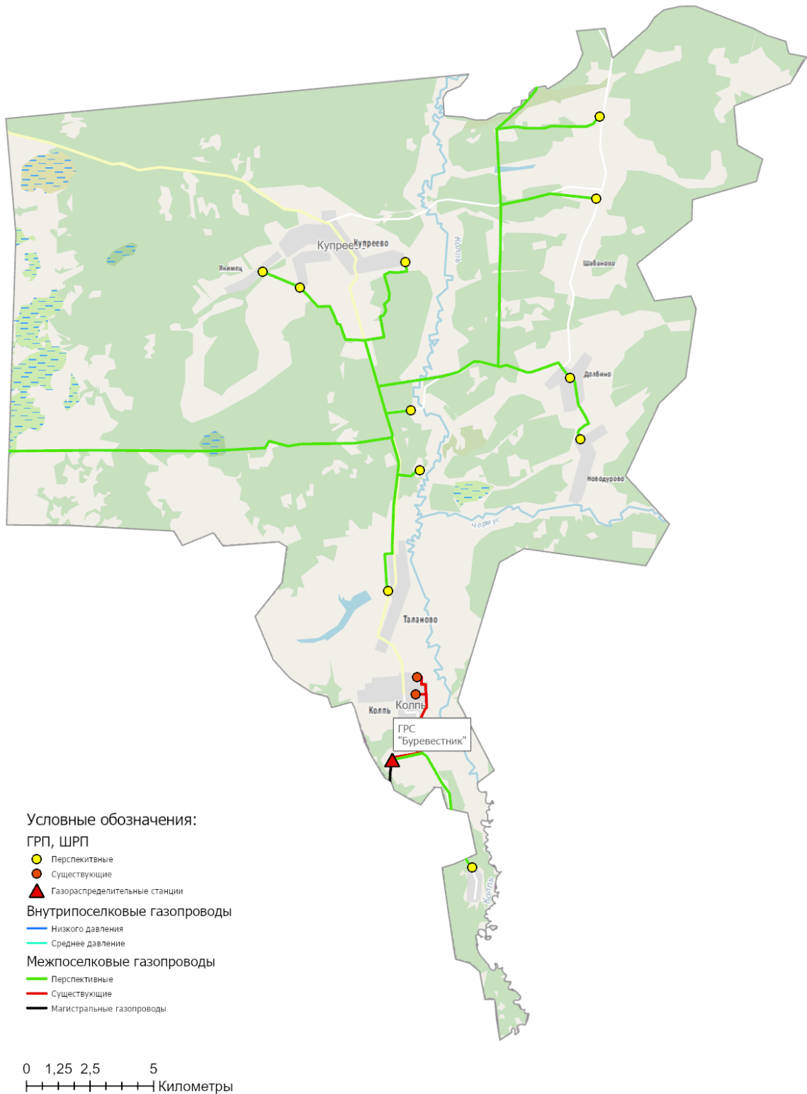
Рисунок 8.5.1 - Перспективная схема газификации территории муниципального образования
