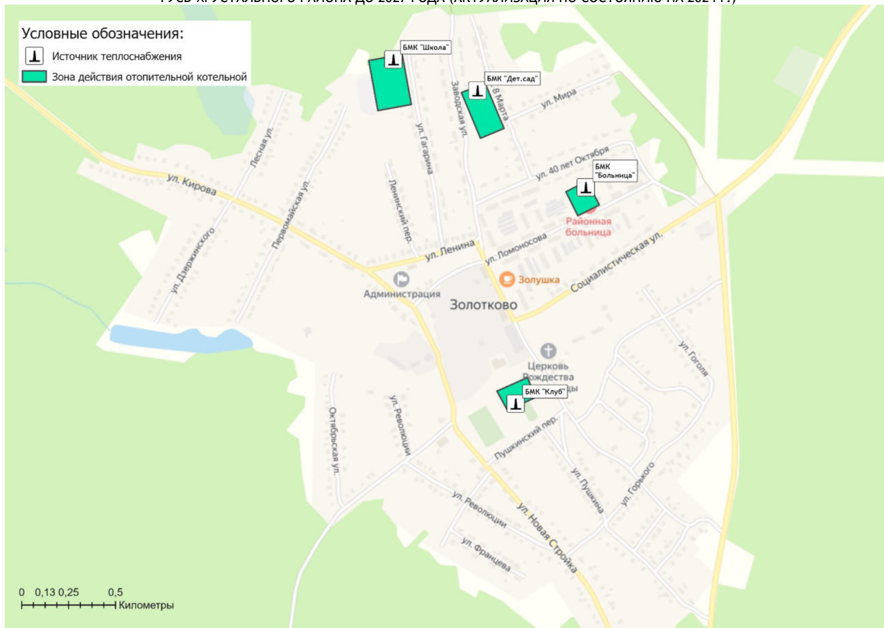
Рисунок 1.4.1 - Зона действия котельной на территории муниципального образования пос. Золотково
