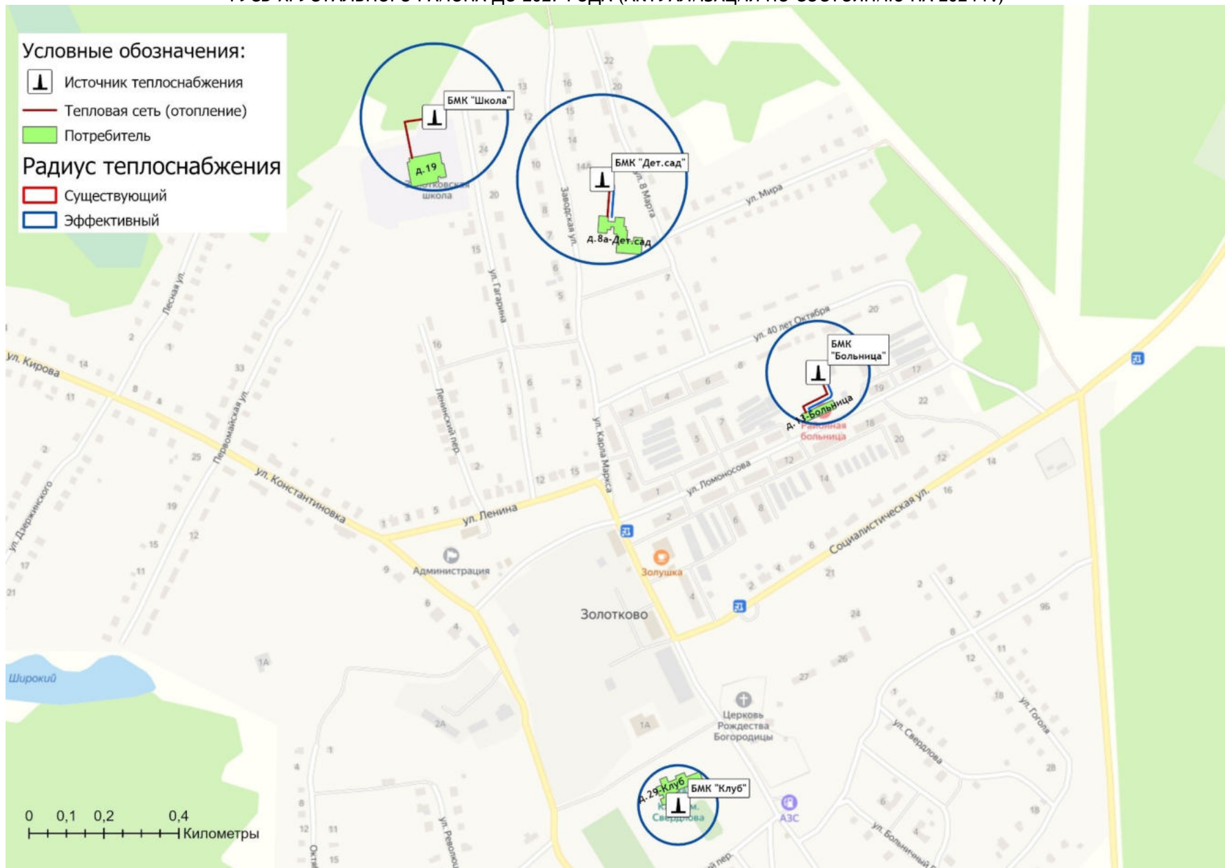
Рисунок 2.5.1 - Радиусы теплоснабжения систем теплоснабжения пос. Золотково
